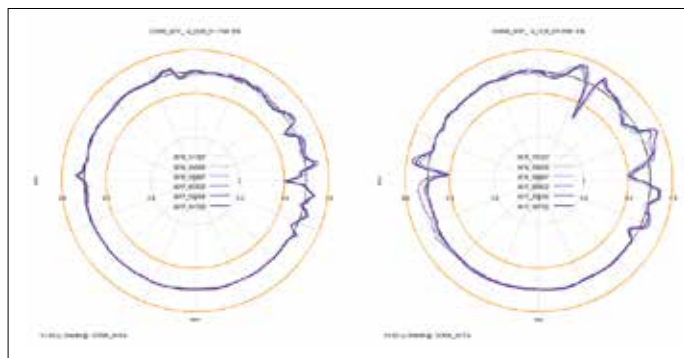
\Delta R der beiden Räder in Polardarstellung. Mehrere Messungen desselben Rades übereinander gelegt zeigt die ausgezeichnete Reproduzierbarkeit. Auch die hohe Auflösung der Ergebnisse ist ersichtlich.
